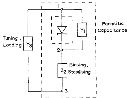
Fig. 3. Amplifier.
